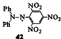
дифенилпикрилгидразил
