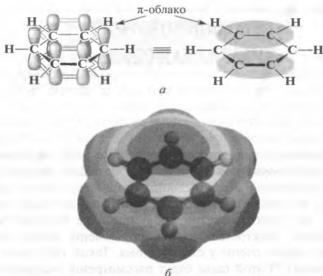
Рис. 2.1. (а) Традиционное изображение перекрывания p -орбиталей, образующих \pi -облако бензола. (б) Карта распределения электростатического потенциала молекулы бензола, на которой видно, что самая высокая электронная плотность находится над шестичленным кольцом и под ним по центру молекулы
