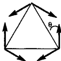
Рис. 4.7. Перекрывание орбиталей в циклопропане. Стрелки направлены к центру электронной плотности
