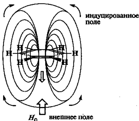
Рис. 2.7. Кольцевой ток в молекуле бензола
