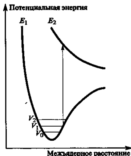
Рис. 7.3. Переход в диссоциативное состояние приводит к расщеплению связи
