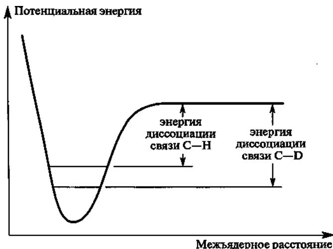
Рис. 6.4. Диаграмма энергии молекулы. Связь C—D имеет более низкую энергию нулевых колебаний и соответственно более высокую энергию диссоциации, чем связь C—H
