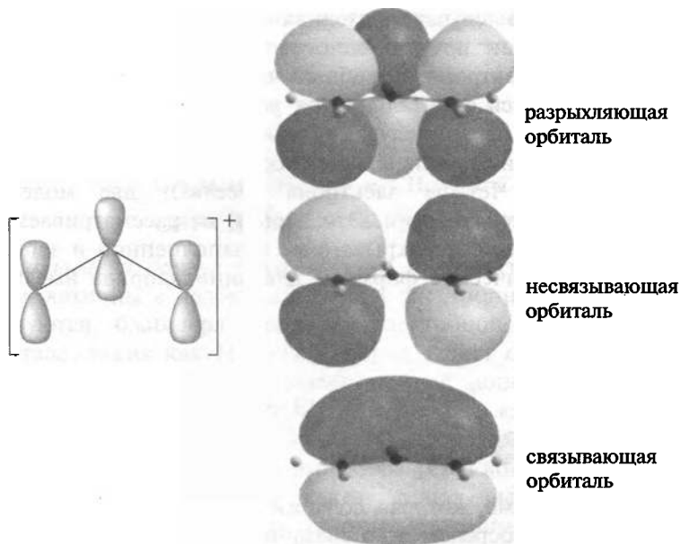
Рис. 2.5. Три орбитали аллильной системы, образованные перекрыванием трех p -орбиталей
