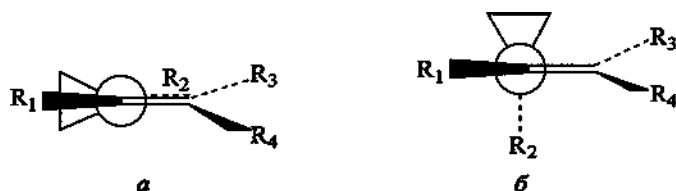
Рис. 4.8. Конформации \alpha -циклопропилалкенов. В конформации a сопряжение максимально, в конформации b — минимально
