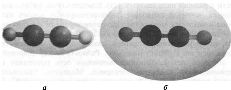
Рис. 1.7. Молекула ацетилена. Обратите внимание на то, что концентрация электронной плотности вдоль линии, соединяющей ядра, согласуется с перекрыванием \sigma -орбиталей в тройной связи (а). Карта электронного потенциала, показывающая места концентрации электронной плотности между атомами углерода, соответствующие двум \pi -связям (б)
