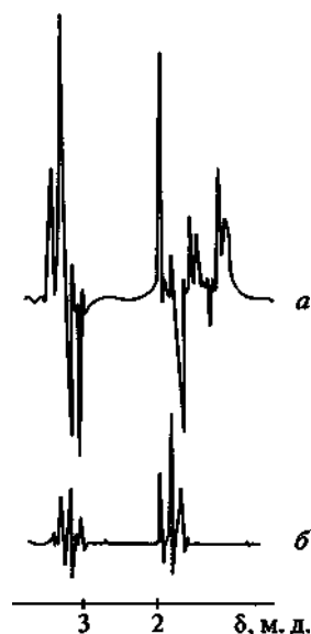
Рис. 5.1. Спектр ЯМР, снятый в процессе реакции между EtI и EtLi в бензоле (а). Область между 2,5 и 3,5 м. д. сканирована с двойной амплитудой. Сигналы при 1,0 и 1,6 м. д. относятся к бутану, некоторое количество которого также образуется в ходе реакции. Эталонный спектр EtI (б). Печатается с разрешения из Ward, H. R.; Lawler, R. G.; Cooper, R. A. J. Am. Chem. Soc. 1969, 91, 746. Copyright © 1969, American Chemical Society
