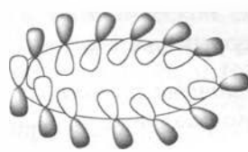
Мёбиус
