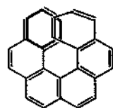
гексагелицен
