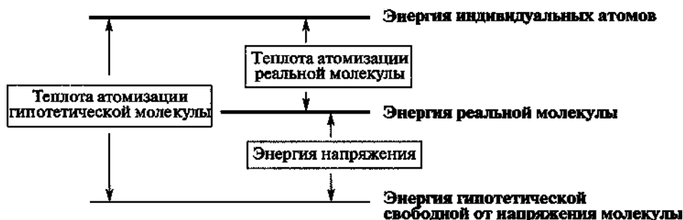
Рис. 4.6. Расчет энергии напряжения
